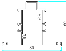
ĐÓ CHIA KHUNG
