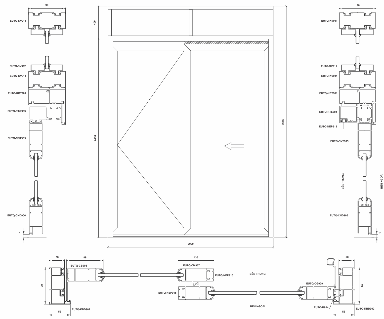
CỬA TRƯỢT QUAY 2 CÁNH MỞ TRONG
