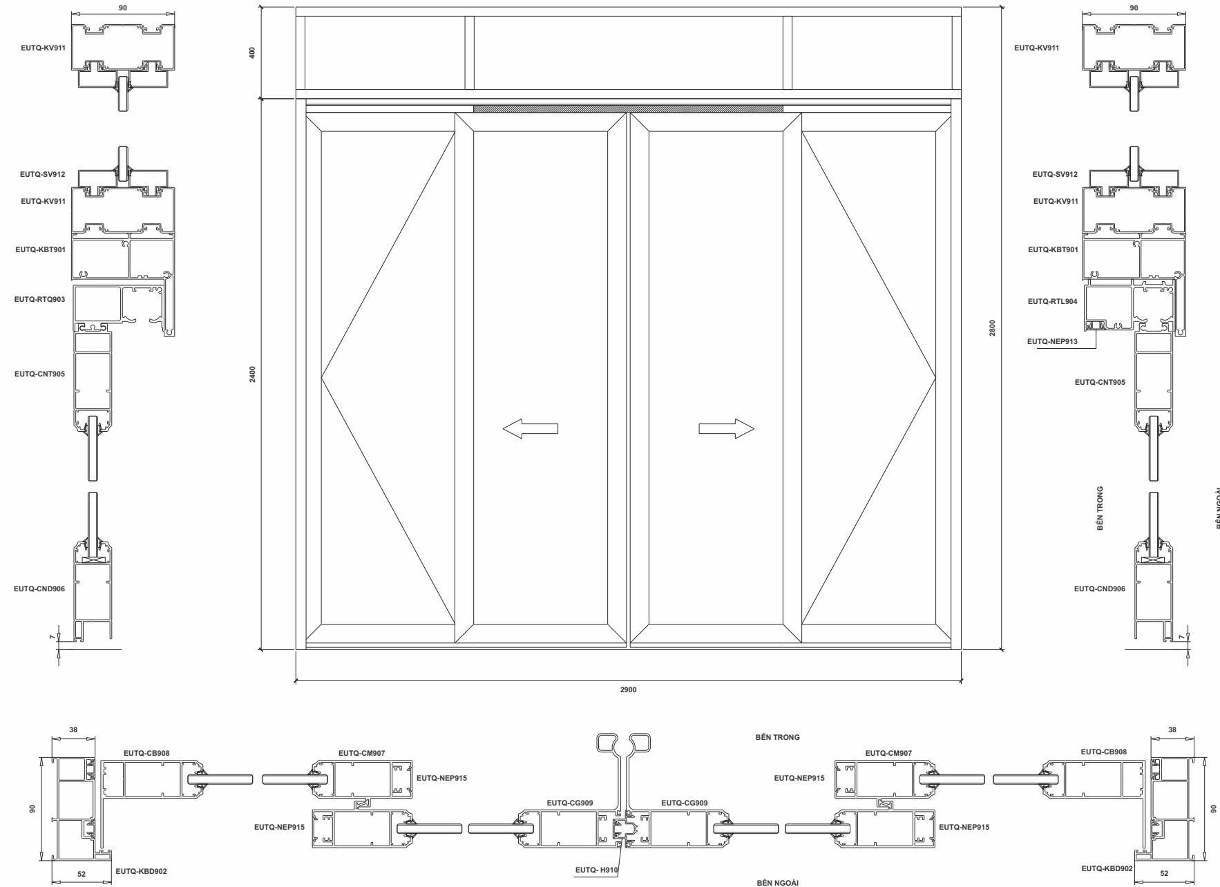
CỬA TRƯỢT QUAY 4 CÁNH MỞ TRONG
