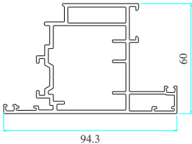
CÁNH ĐI MỞ NGOÀI
