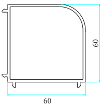
THANH CHUYỀN GÓC 90
