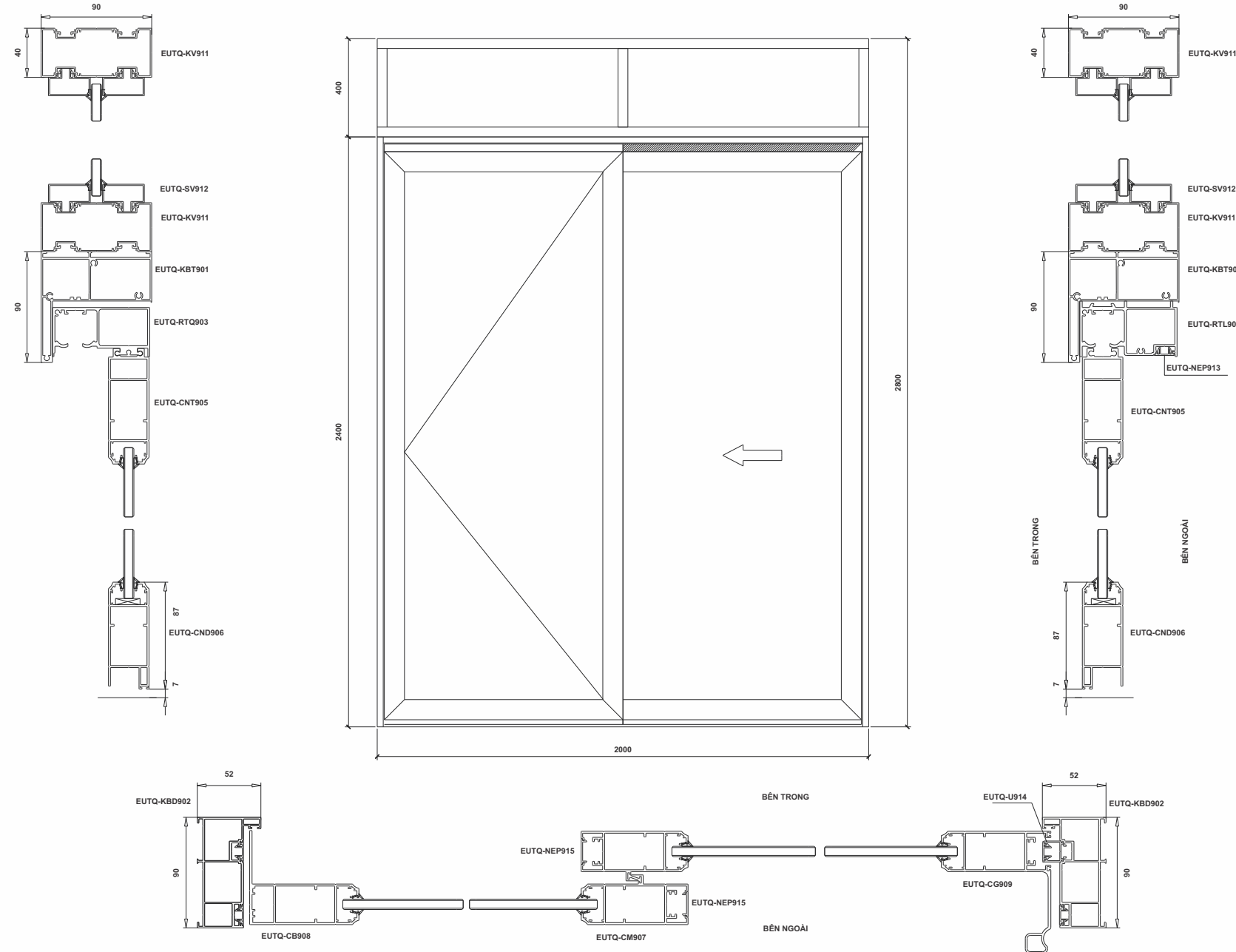
CỬA TRƯỢT QUAY 2 CÁNH MỞ NGOÀI
