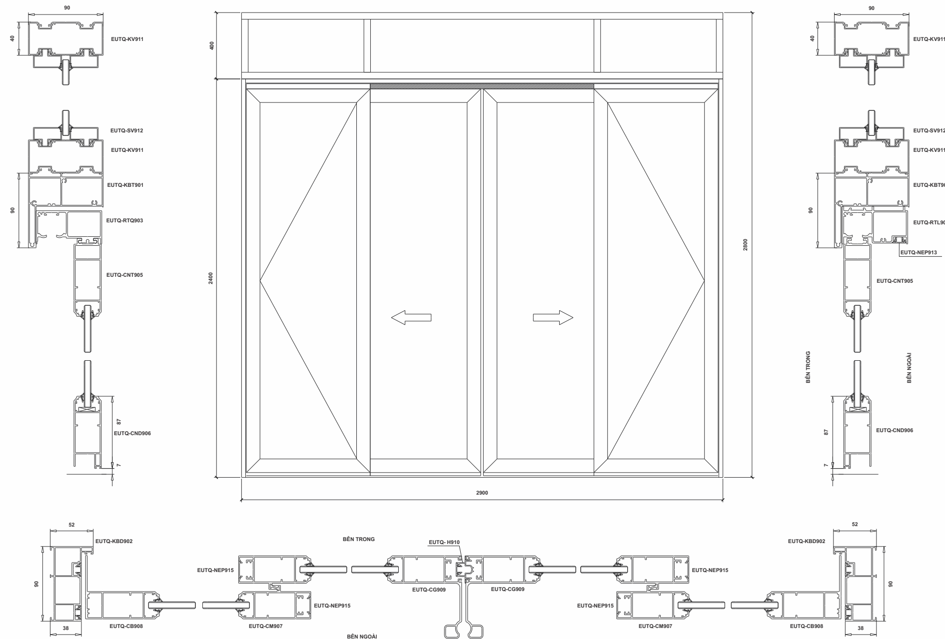
CỬA TRƯỢT QUAY 4 CÁNH MỞ NGOÀI
