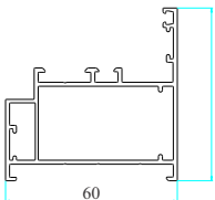
KHUNG BAO CỬA SÒ
