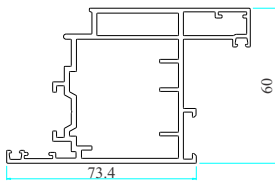
CÁNH CỬA ĐI MỞ TRONG
